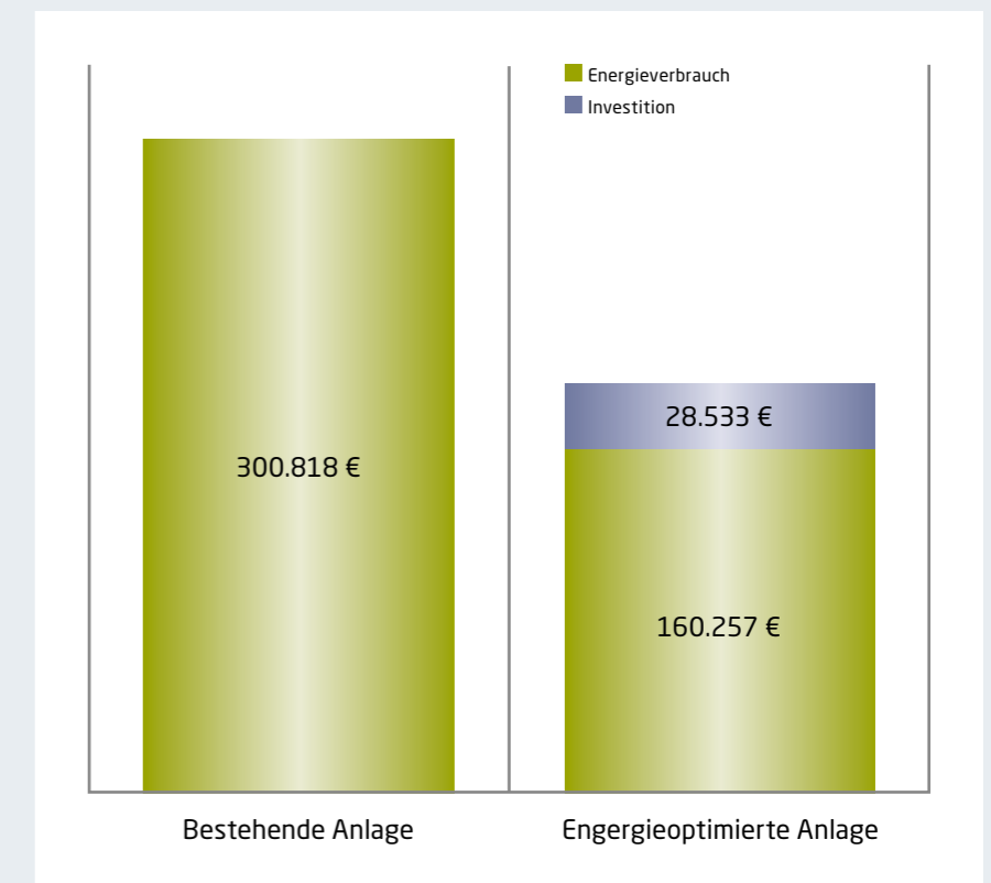
Vergleich der Betriebskosten und Investitionskosten einer Anlage mit 3 Umluftkühlgeräten zur Klimatisierung eines Rechenzentrums - vor und nach einer Umrüstung der Ventilatoren.
