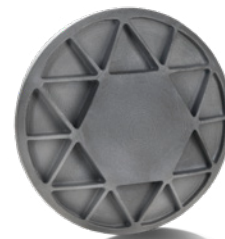
^ 3D-gedruckter Spiegel für optische Systeme in Satelliten
