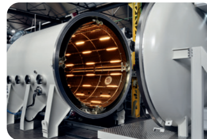
^ Temperatur-Vakuumkammern zum Testen von Raumfahrt-ausrüstung
