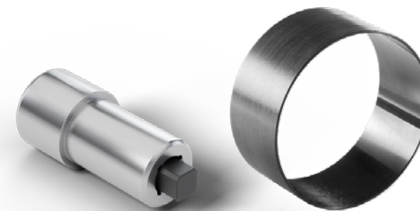
^ Wellenerder für Öllauf & Armierungshülse zur Rotorstabilisierung
